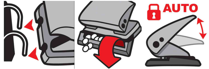
Anschlagsschiene - System zum Zentrieren - Entleerungsklappe - Oberteilverriegelung
