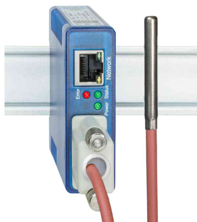
Symbolbild: Anwendung Web-Thermometer, PT-100/PT-1000
