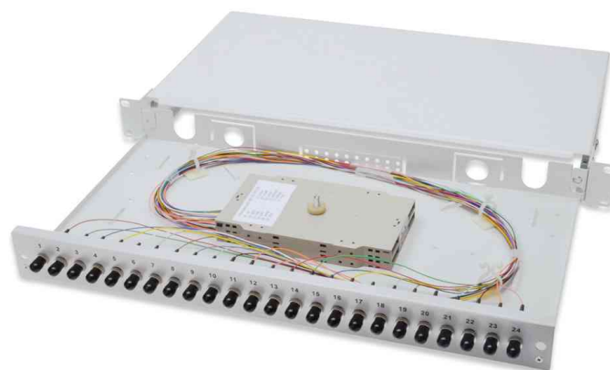
19" Glasfaser LWL Spleißbox, 24 x ST
