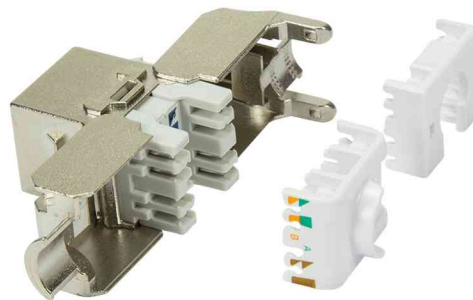
Keystone Modul Kat.6A, geschirmt, Detailansicht
