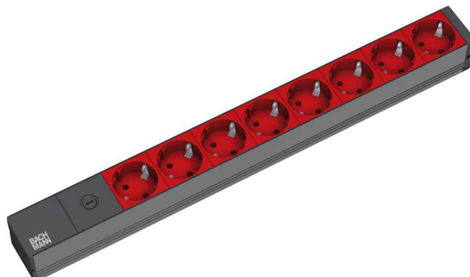
19" Steckdosenleiste, schwarz / rot
