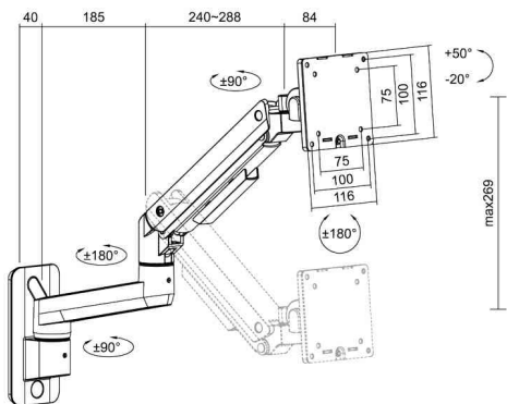
Monitorarm zur Wandmontage, Abmessungen
